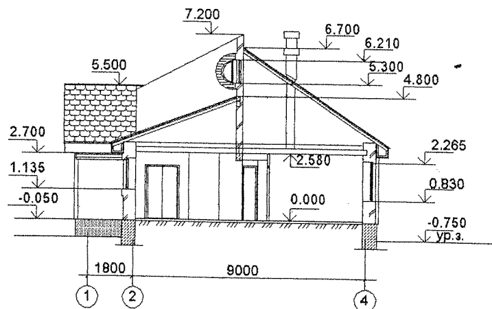
РАЗРЕЗ 1-1
