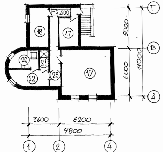
ПЛАН ПОДВАЛА.
