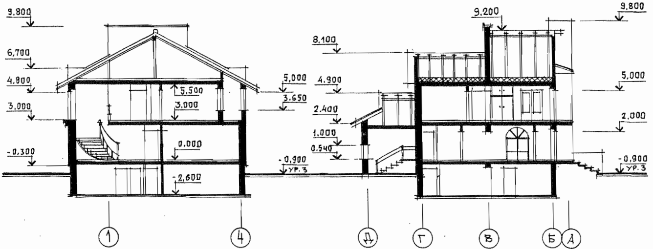
РАЗРЕЗ 2.2
