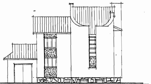
ФАСАД А-А
