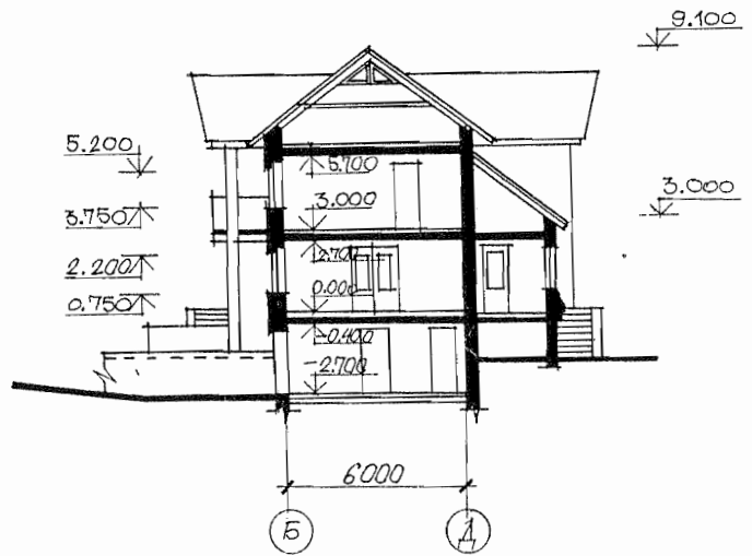
РАЗРЕЗ 1-1
